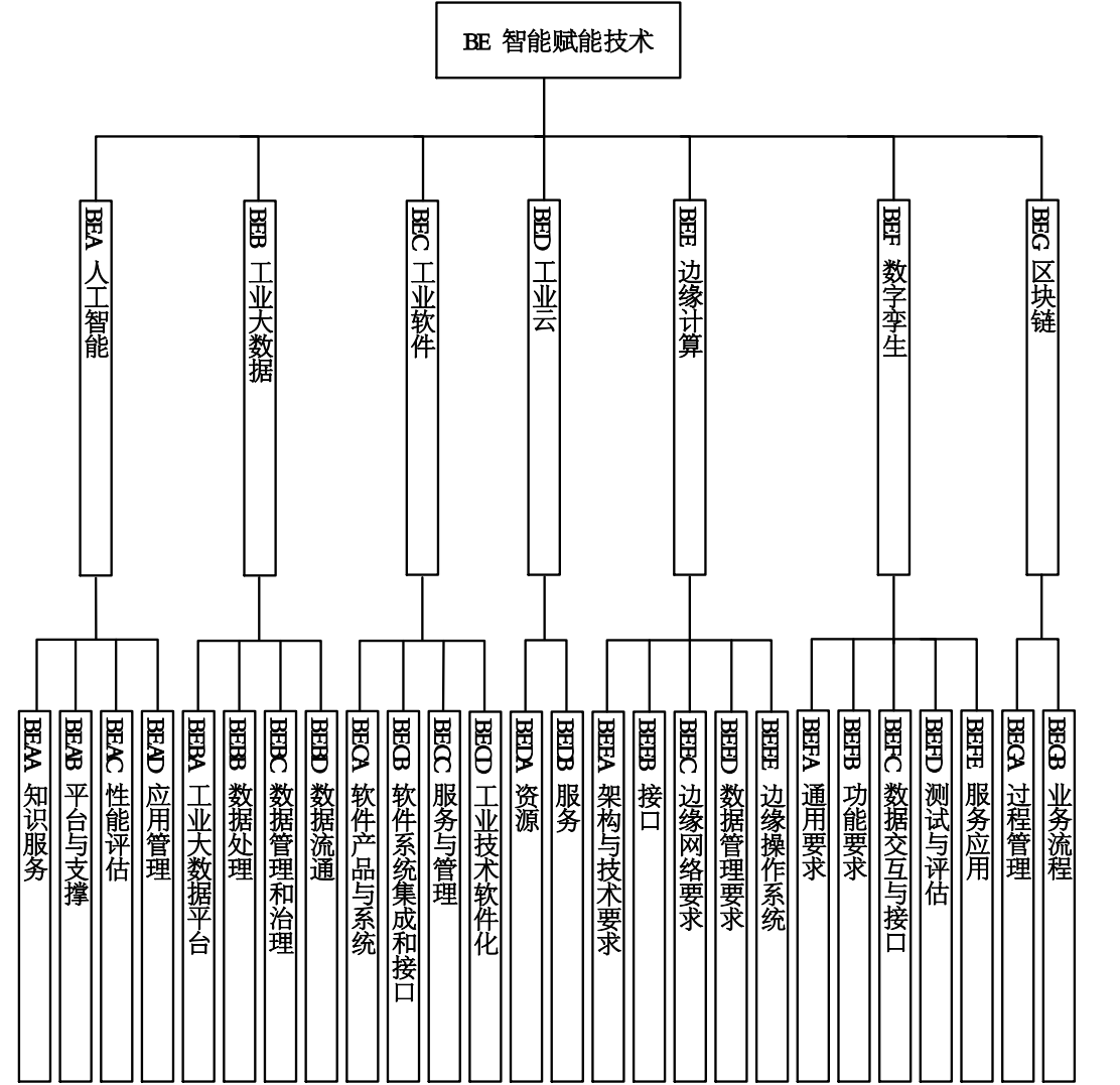
图 9 智能赋能技术标准子体系
