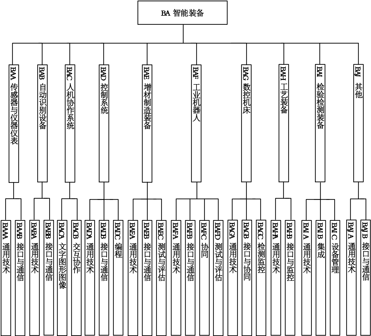
图 5 智能装备标准子体系
